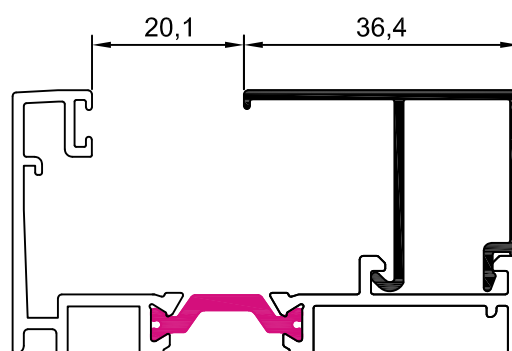
10010 junquillo 36,4 mm
