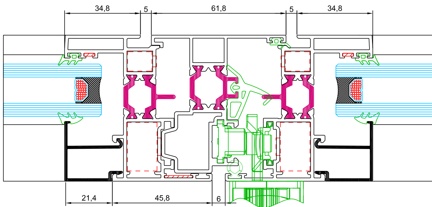
sección 5
