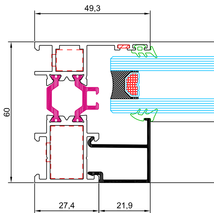
sección 1
