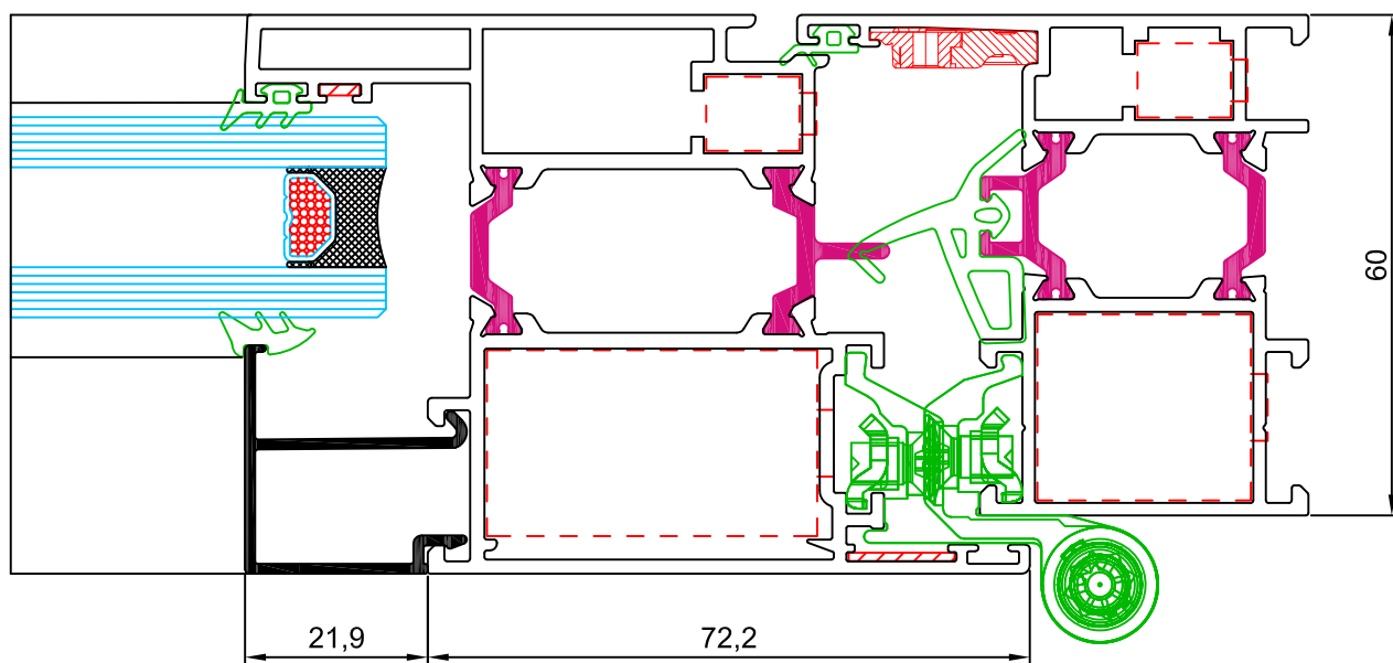
sección 7
