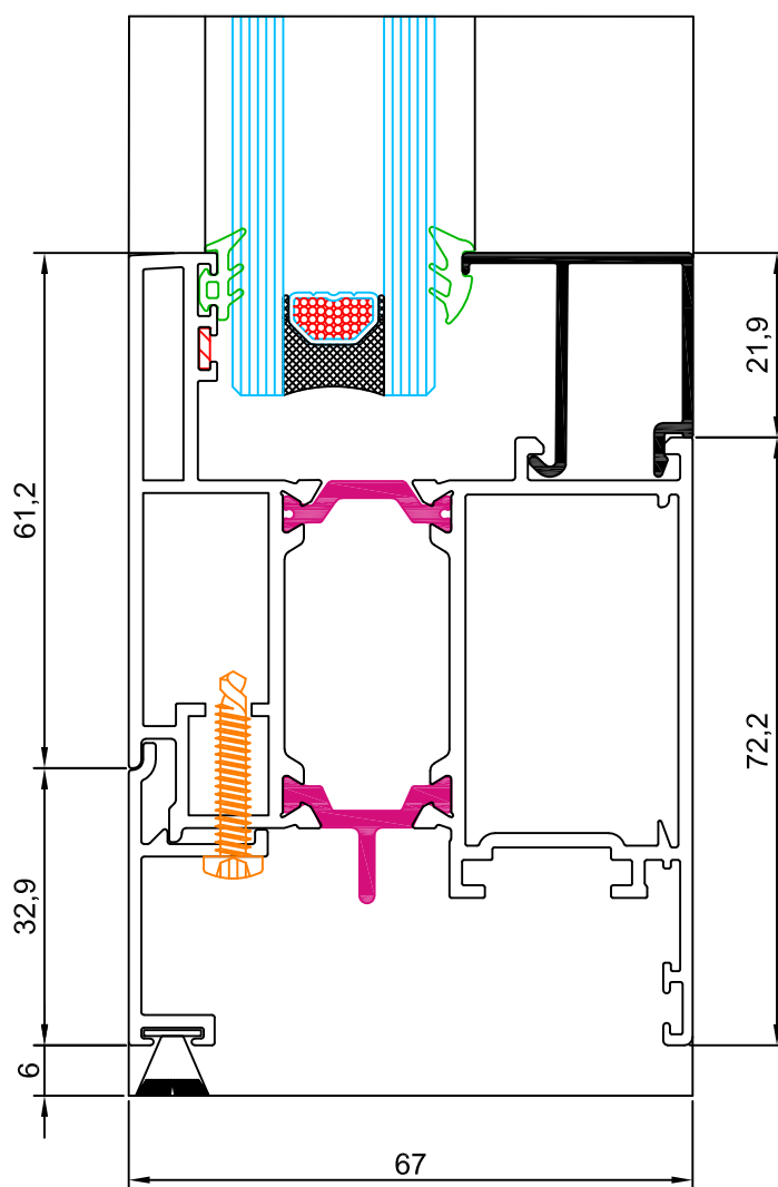
sección 9
