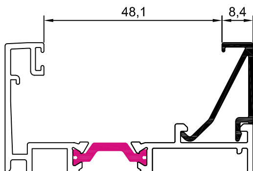
10001 junquillo 8,4 mm
