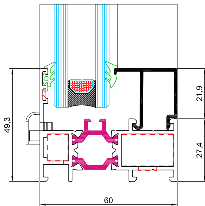
sección 2
