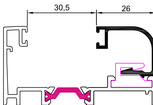
12004 junquillo 26 mm
