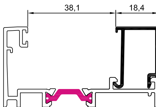
10004 junquillo 18,4 mm
