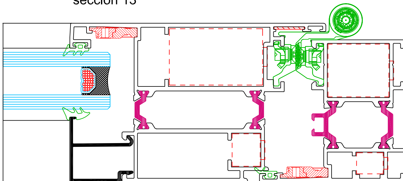
sección 13
