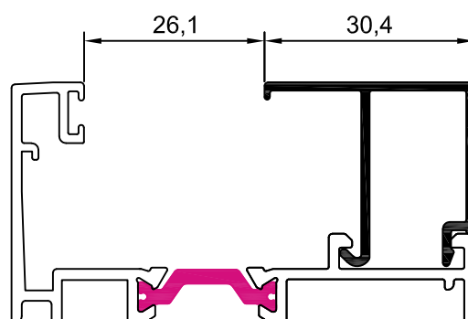
10008 junquillo 30,4 mm
