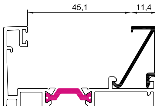
10002 junquillo 11,4 mm
