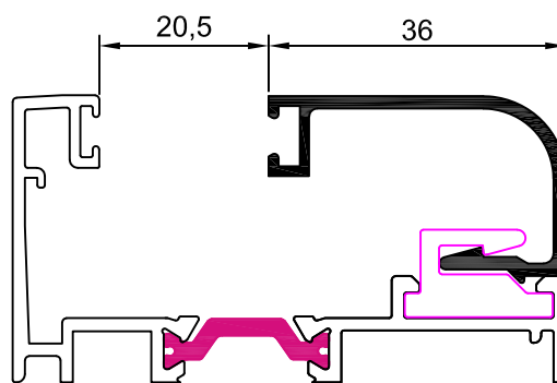
12006 junquillo 36 mm
