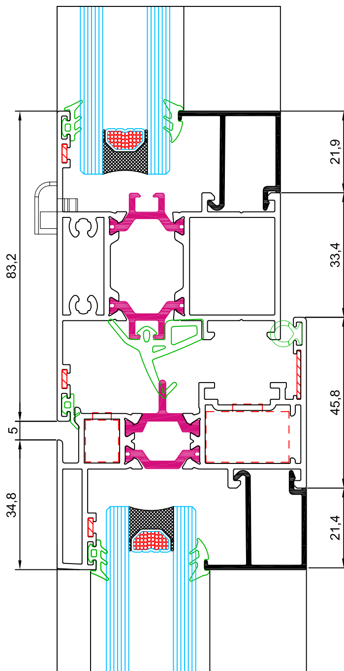
sección 6
