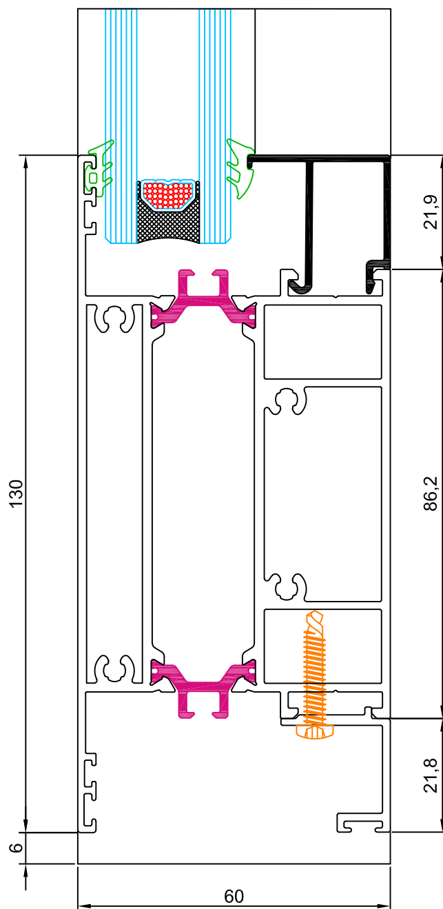
sección 15
