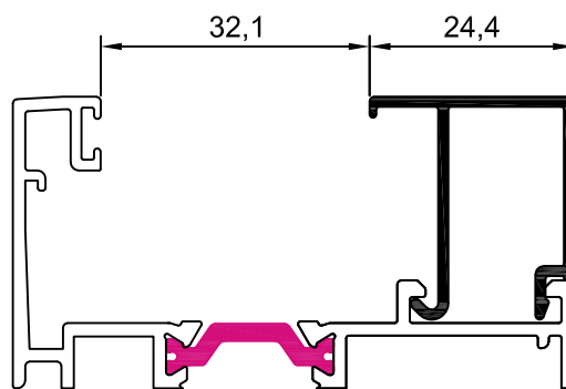
10006 junquillo 24,4 mm
