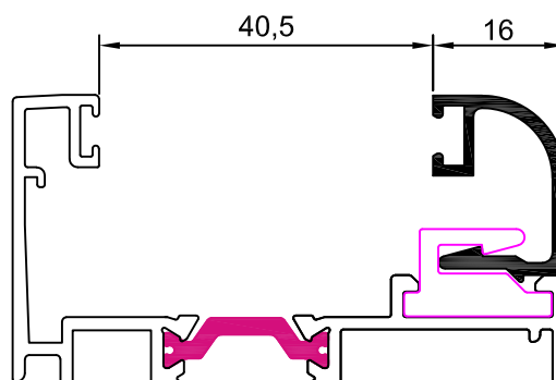
12002 junquillo 16 mm
