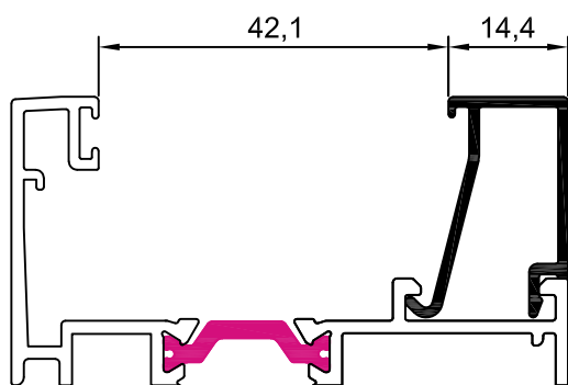
10003 junquillo 14,4 mm
