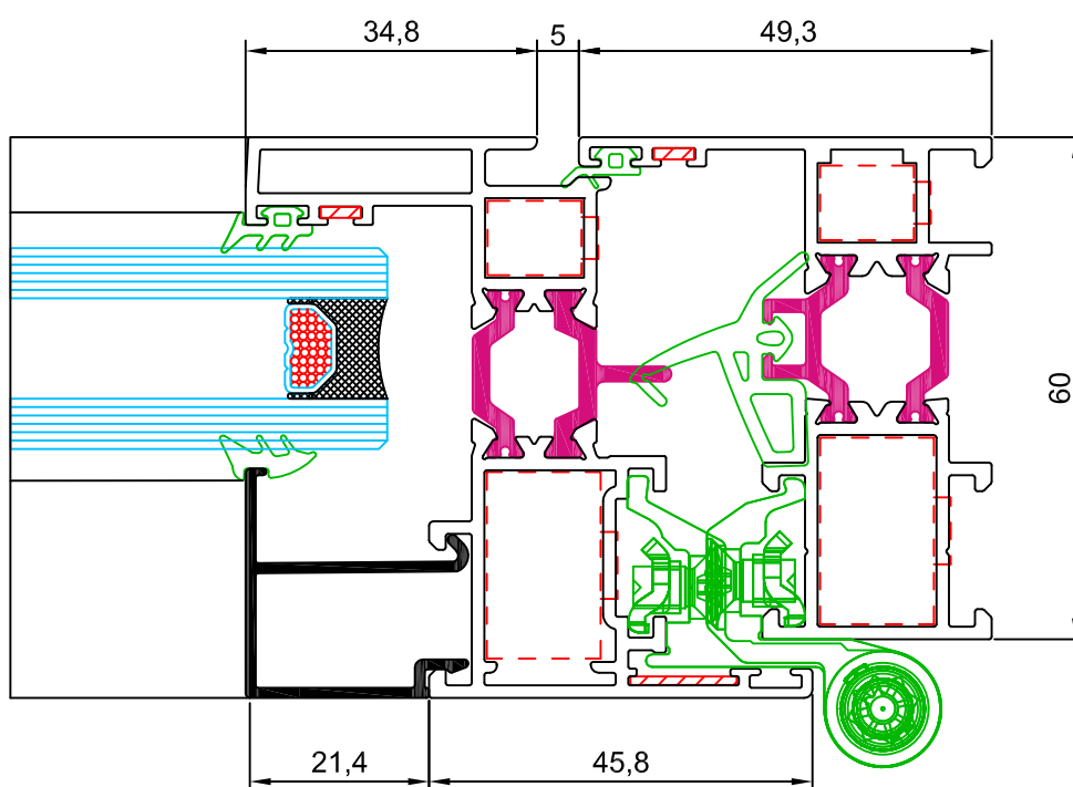
sección 3
