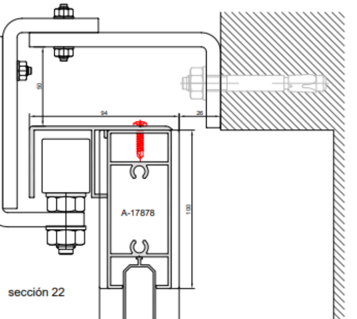
escala 0.75:1
