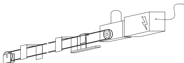
FE 053.120 - Kit Motorización TIPO 3 hasta 12 m
