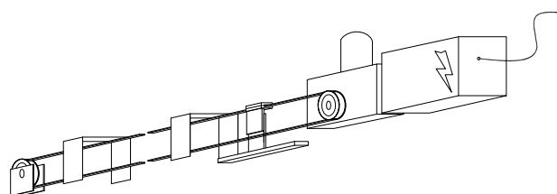
FE 054.120 - Kit Motorización TIPO 4 hasta 12 m
