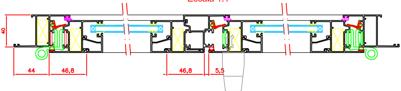
Sección Horizontal A - A' Escala 1:1
