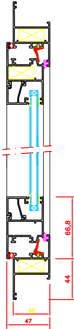
Sección Vertical B - B' Escala 1:1
