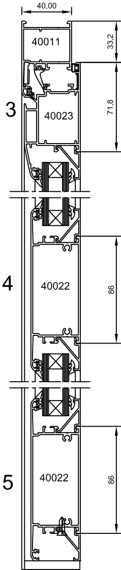
Escala Sección 1:3
