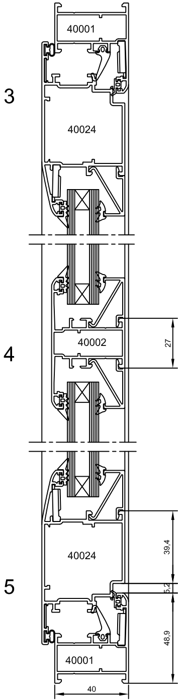
1 Escala Sección 1:2
