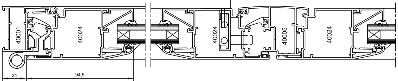
1 Escala Sección 1:2
