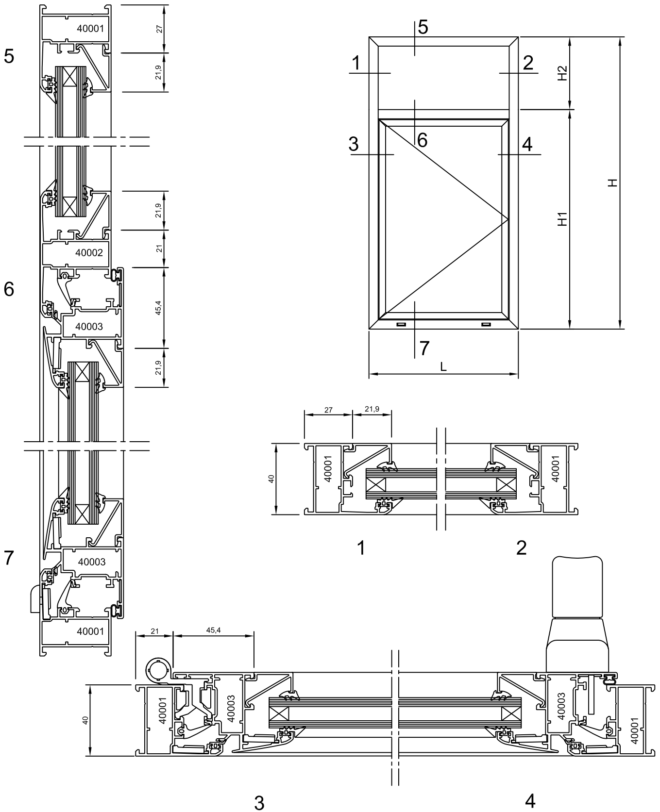
Escala Sección 1:2
