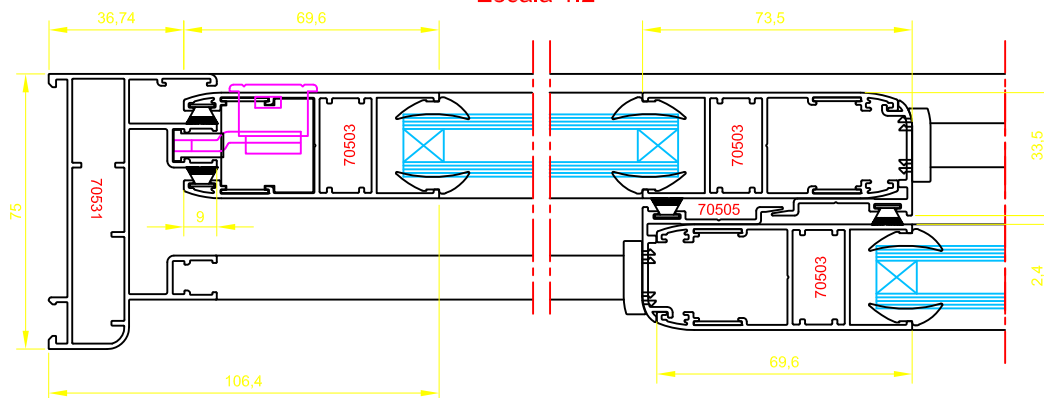
Sección Horizontal A-A' Escala 1:2
