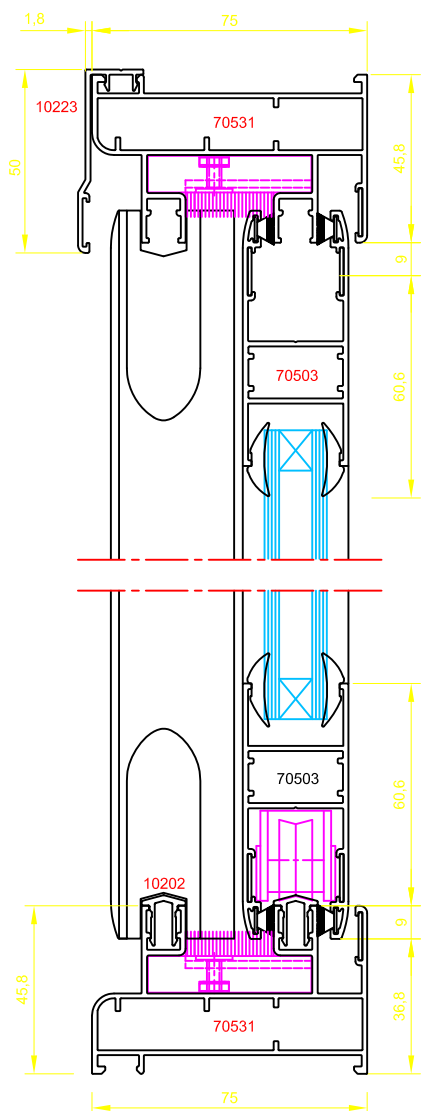
Sección Vertical B-B' Escala 1:2
