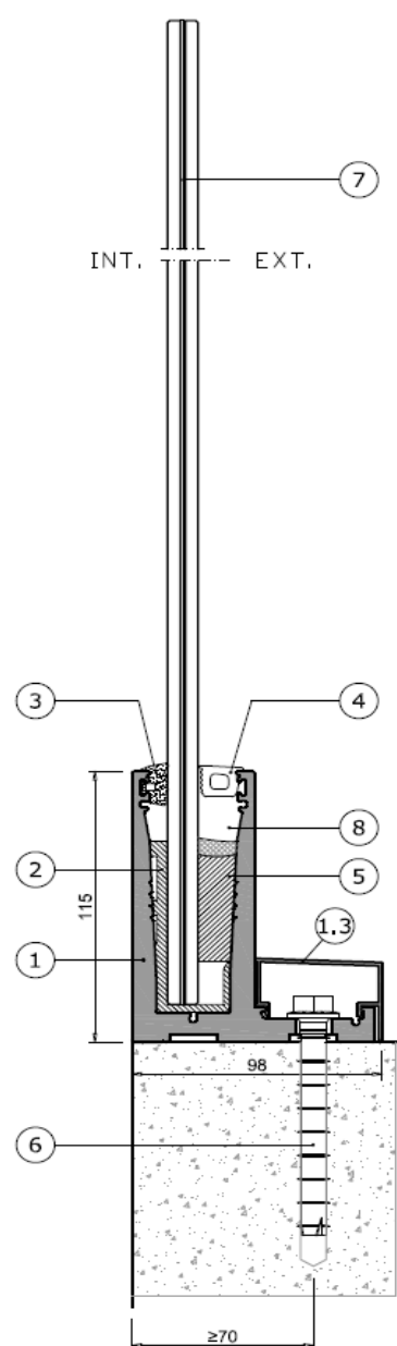
SECCION A-A
